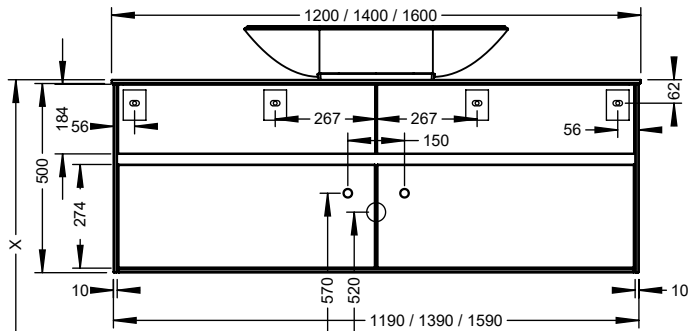
SGAZ120, SGAZ140, SGAZ160 \pm 0 \nabla X = abhängig vom Waschtisch
